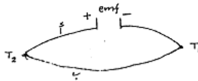
شكل ٢ قوة الدفع الكهربائية في المزدوجة
