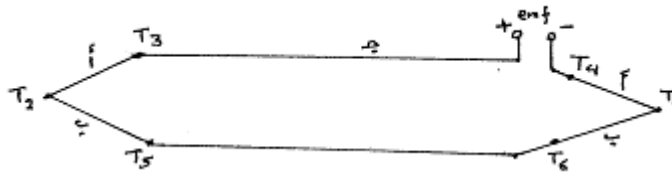
شكل ٣ توصيل المزدوجة الحرارية لمعايرتها
